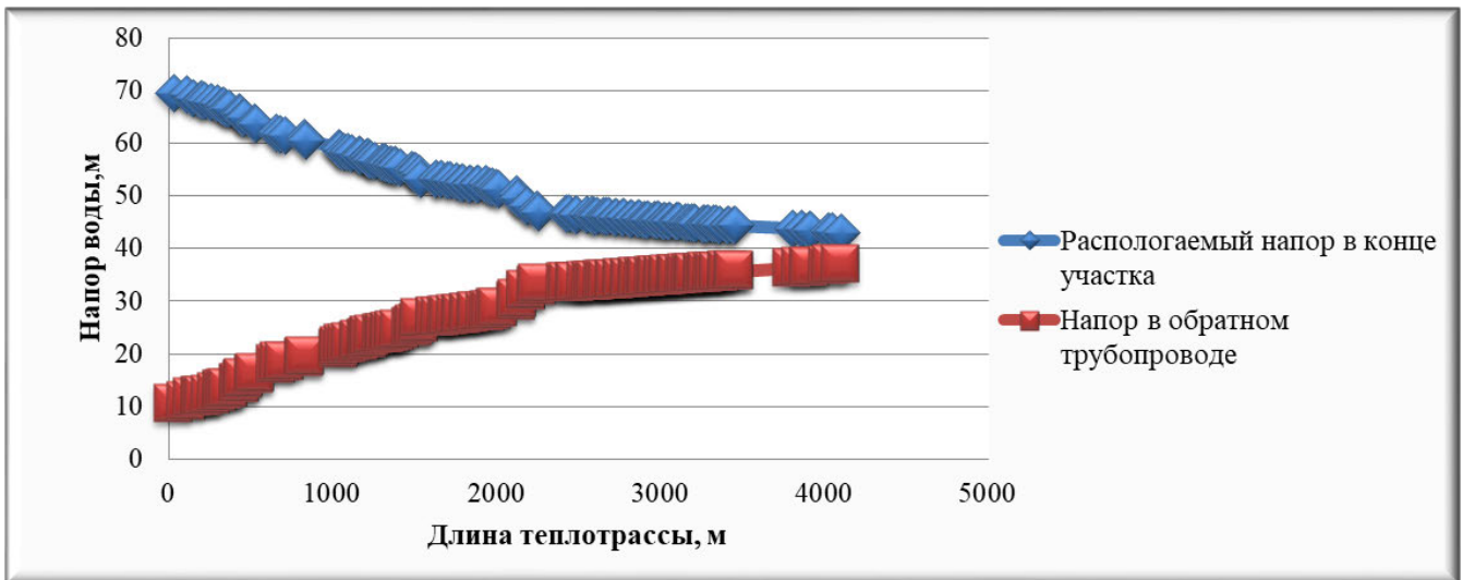
Рисунок 2.5 – Пьезометрический график тепловой сети котельной №1 с. Частоозерье по магистральному выводу
