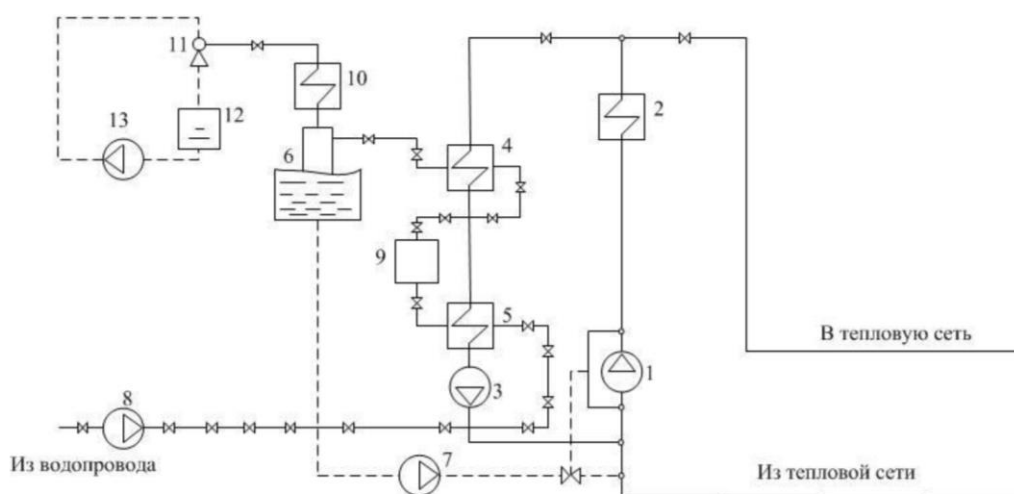
Рисунок 2.3 – Принципиальная тепловая схема котельной с водогрейными котлами: 1 - сетевой насос; 2 - водогрейный котел; 3 - рециркуляционный насос; 4 - подогреватель
