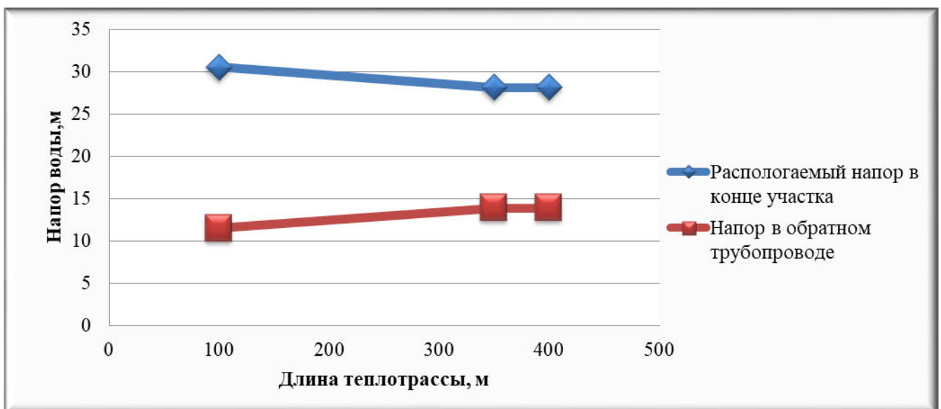
Рисунок 2.6 – Пьезометрический график тепловой сети котельной №2 с. Частоозерье по магистральному выводу
